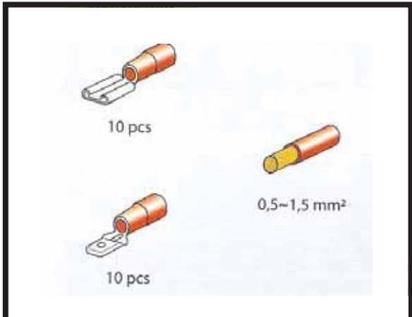
REF. 6445071 JUEGO TERMINAL MACHO RJ 10 U. 6.3X8MM
