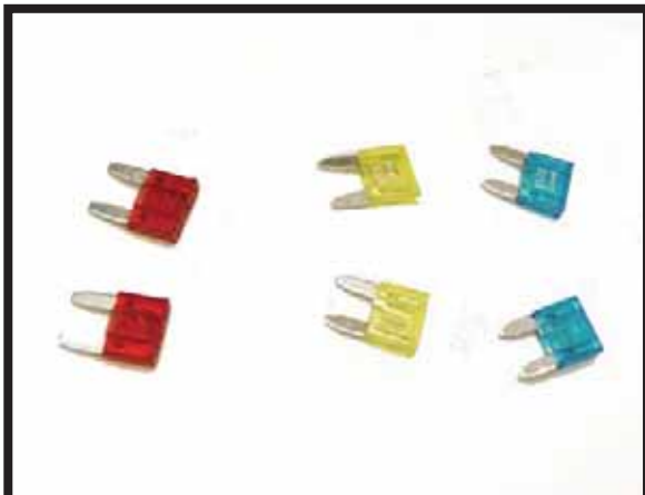
FUSIBLE MINI 3-4-5-7,5-10-15-20-25-30 AMP
