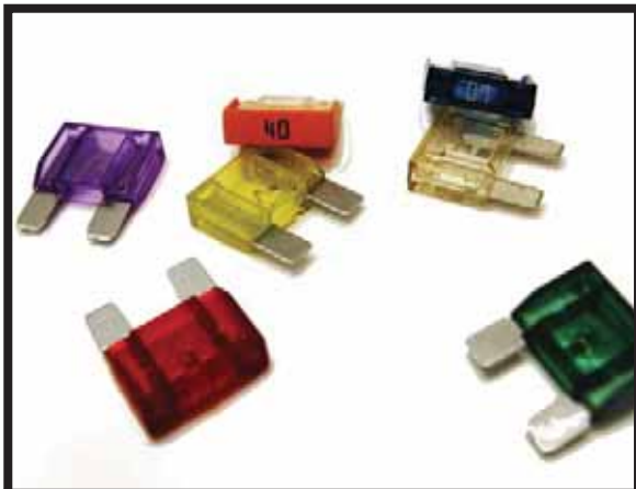
FUSIBLE MAXI 20-30-40-50-60-70-80 Y 100 AMP
